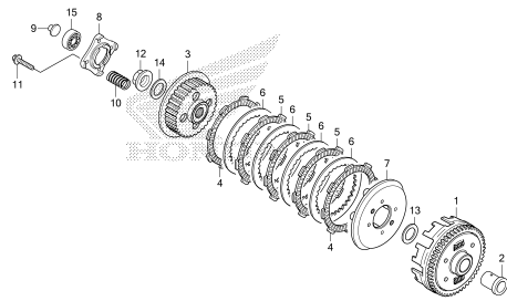
CLUTCH
